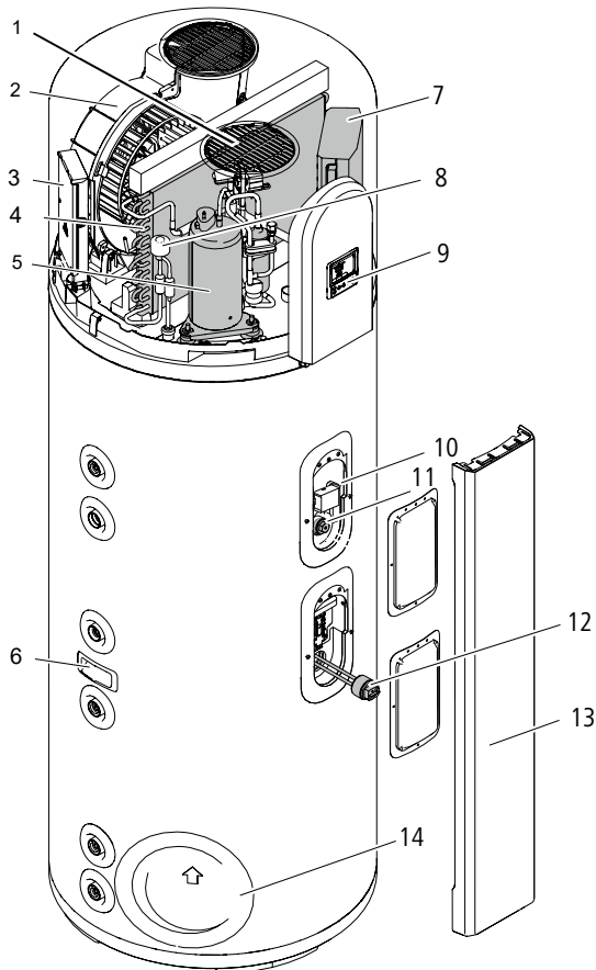
Abb. 1: Komponenten
