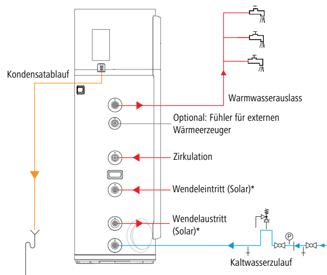
Abb. 5: Anschlussbild
